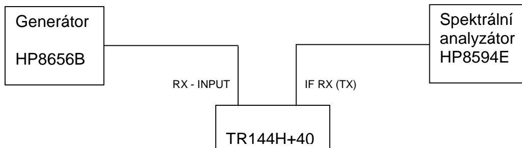
obr.č.4 Blokové schéma zapojení
