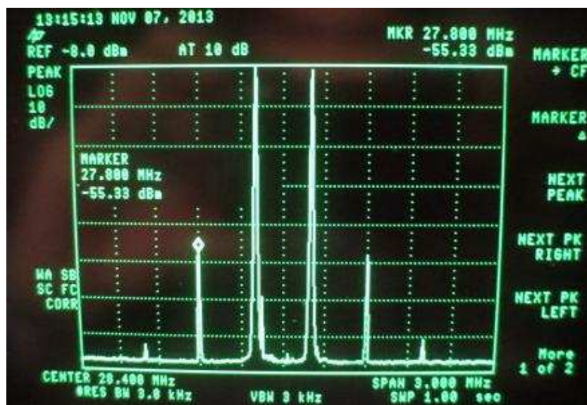
obr.č.13 Výstupní signál z transvertoru při vstupním signálu -15\text{dBm} (na vstupu spektrálního analyzátoru je zařazen 20dB útlum)
